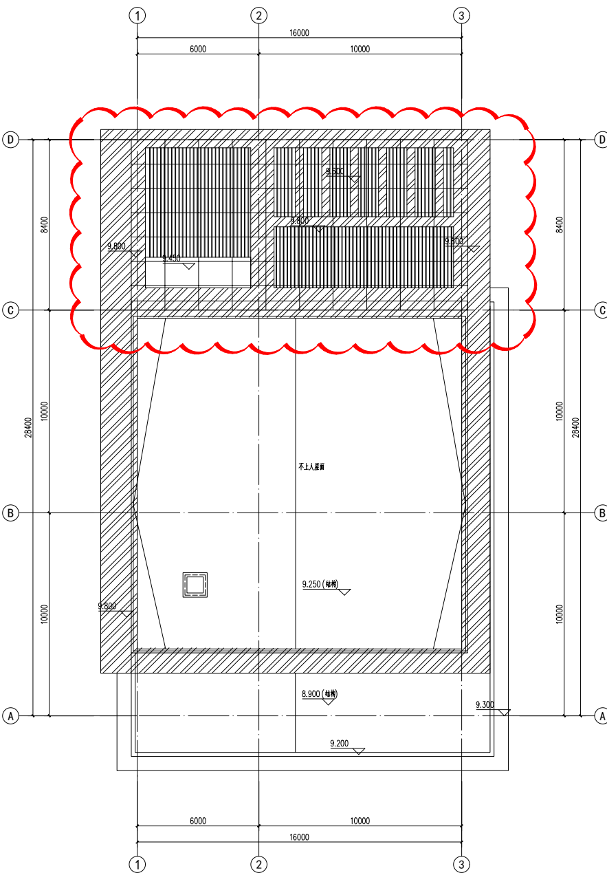
13#楼屋顶平面图（变更后）
