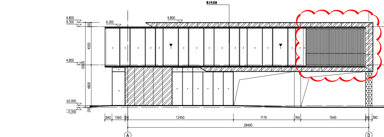
13#楼东立面图（变更后）
