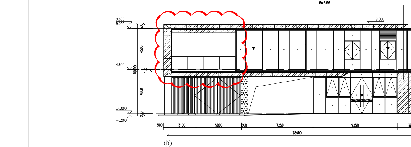
13#楼西立面图（变更前）
