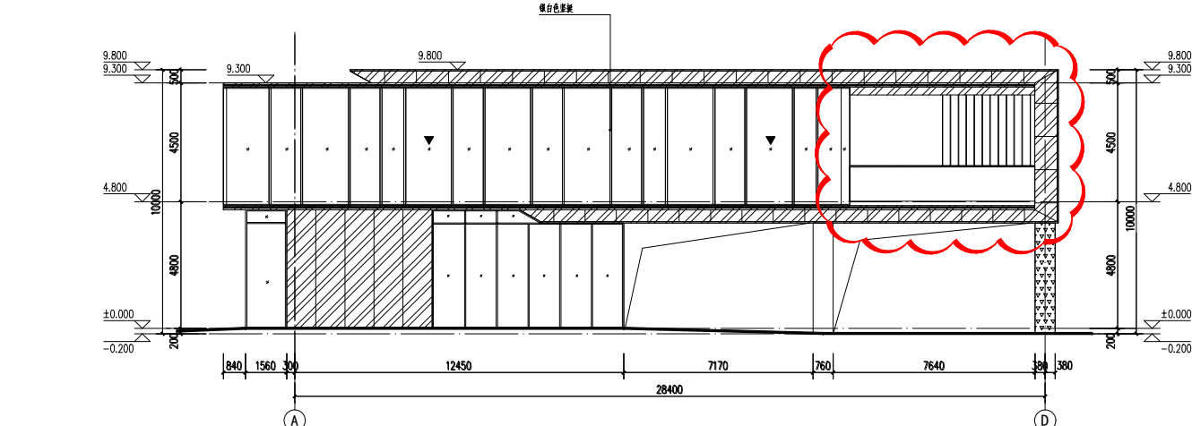
13#楼东立面图（变更前）
