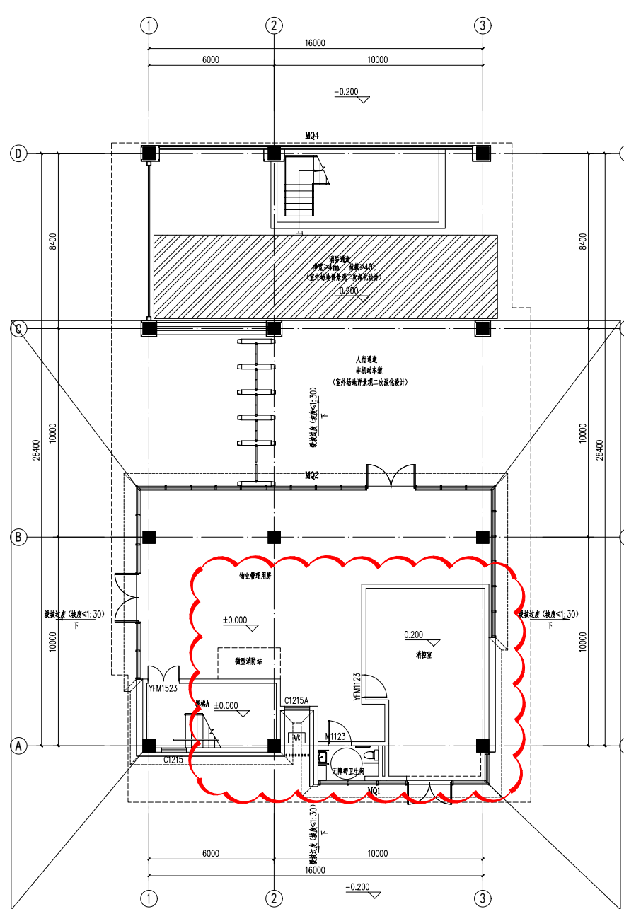
13#楼一层平面图（变更后）
