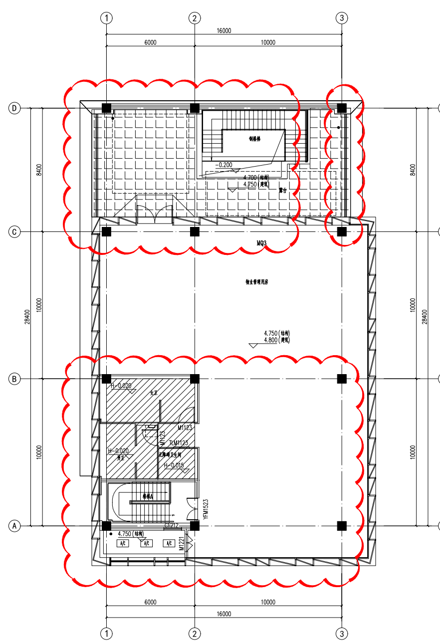
13#楼二层平面图（变更前）
