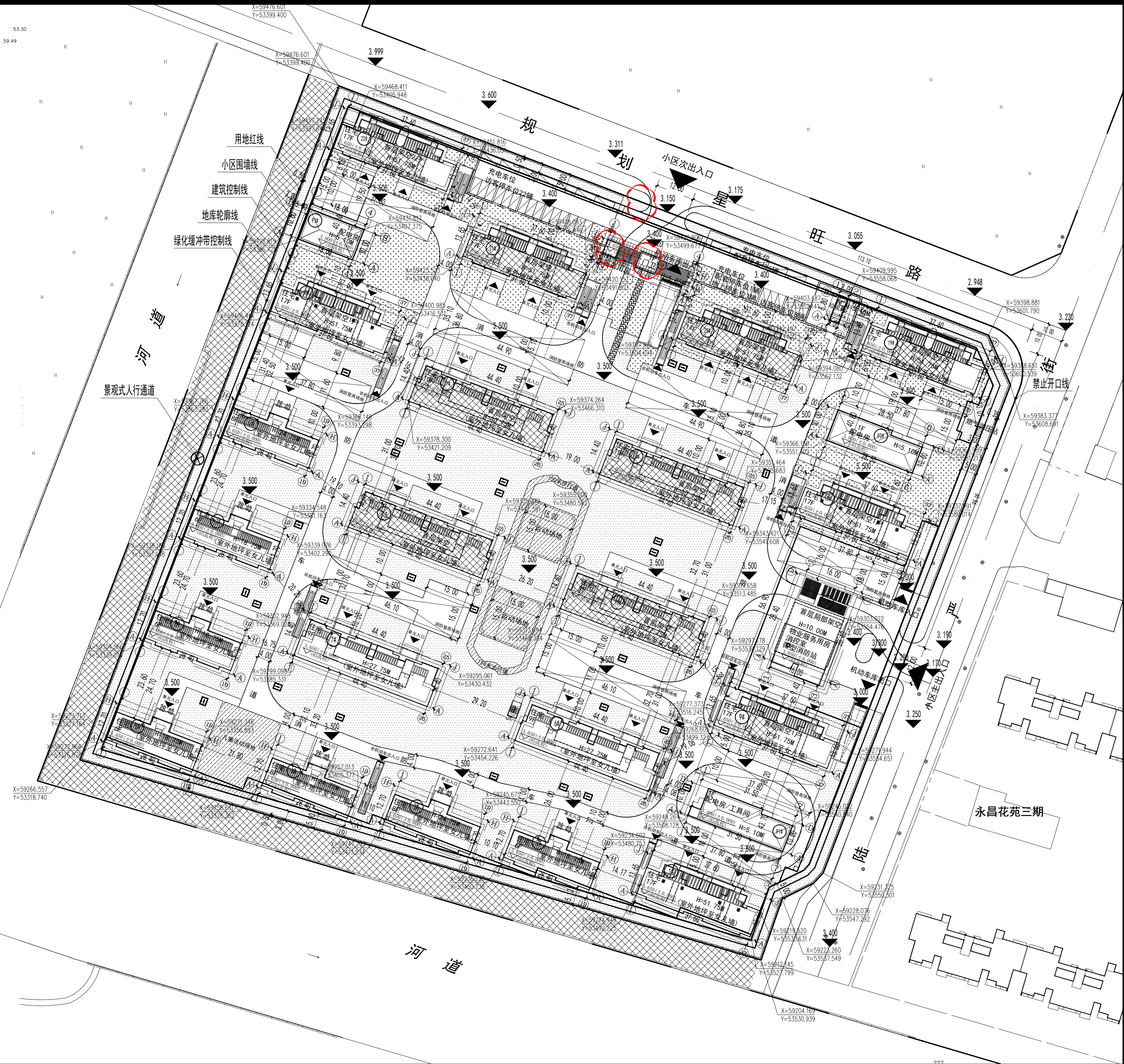
总平面图（变更后）
