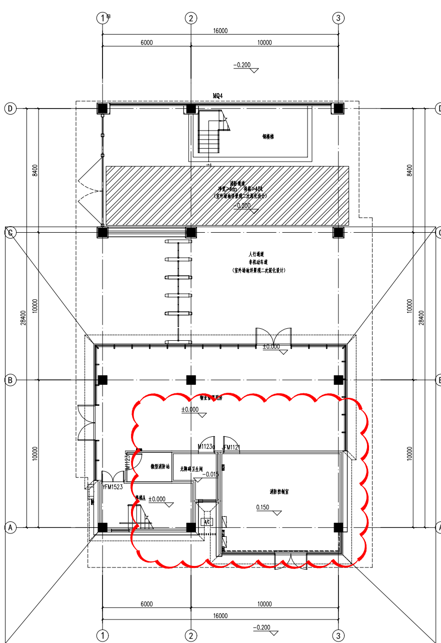
13#楼一层平面图（变更前）
