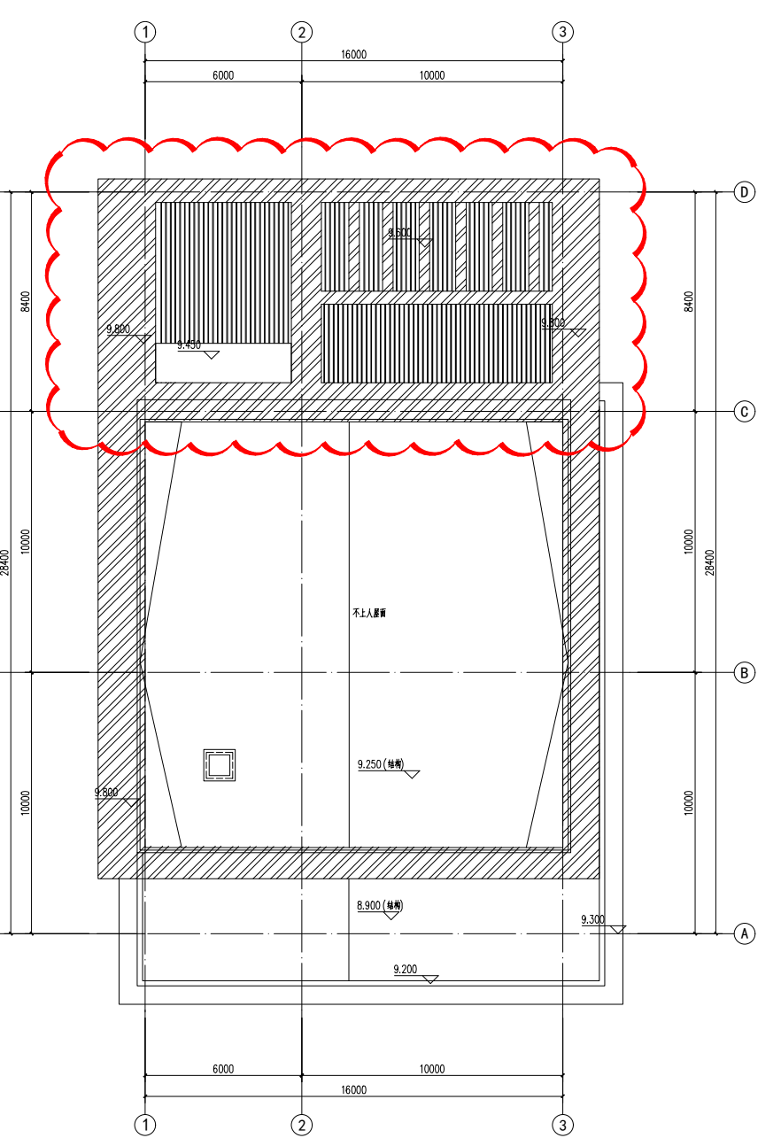
13#楼屋顶平面图（变更前）
