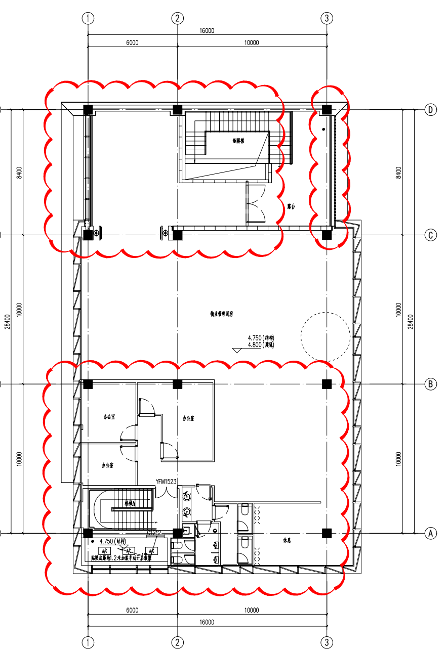
13#楼二层平面图（变更后）
